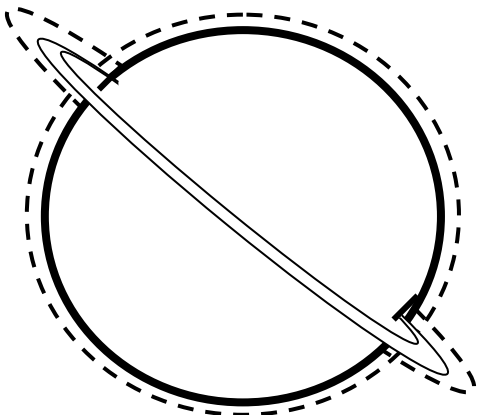
Uranus
